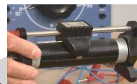
رئوستا یا مقاومت متغیر، معمولاً به طور متوالی در مدار قرار می گیرد
